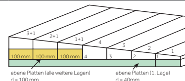
Unterlegung mit Flachplatten, d = 25 bis 160 mm
