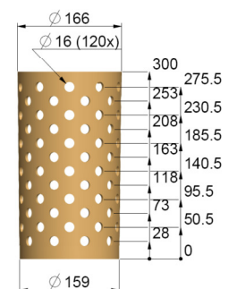
430636 Ställbar inre ring 300 mm hög
