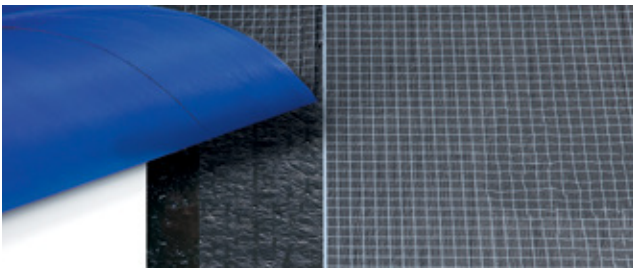
Der Nahtbereich mit Längsrandperforation an der Unterseitenfolie und oberseitiger Hilfslinie für die Nahtüberdeckung.
